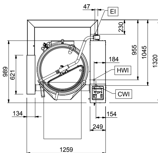
Boven aanzicht
